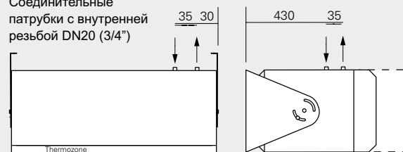
Рис 3: Выходы патрубков теплообменника завес WAC300/400 находятся справа на верхней панели
