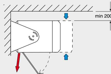
Рис 1: Минимальные расстояния
